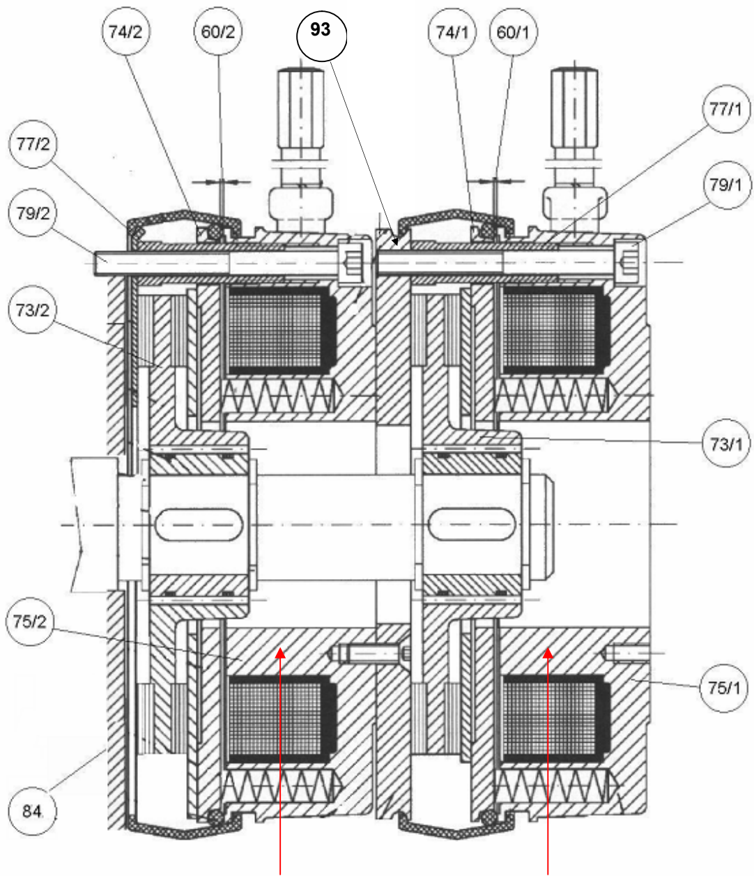
Brake assembly N. 2
